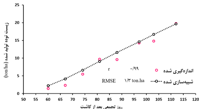
شکل ۵- مقادیر زیست توده تولید شده در مزرعه و شبیه‌سازی شده توسط نرم‌افزار Figure 5- Amounts of biomass produced in the farm and simulated by software
