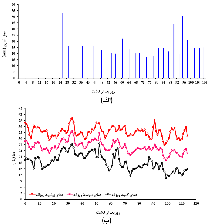
شکل ۲- نمودار آبیاری (الف) و تغییرات دما در طول فصل رشد (ب)
