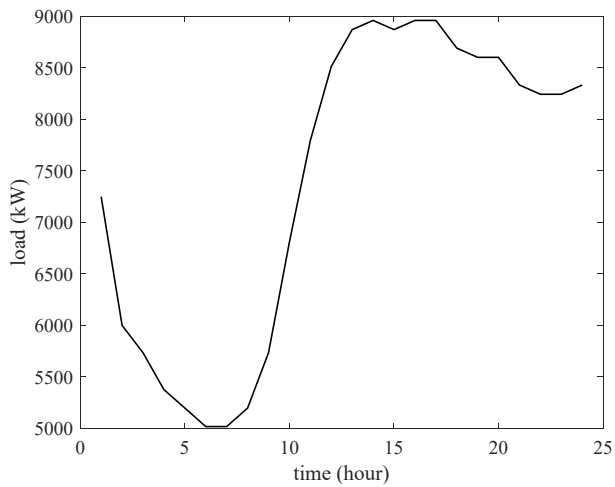
Fig. 9. Hourly load
