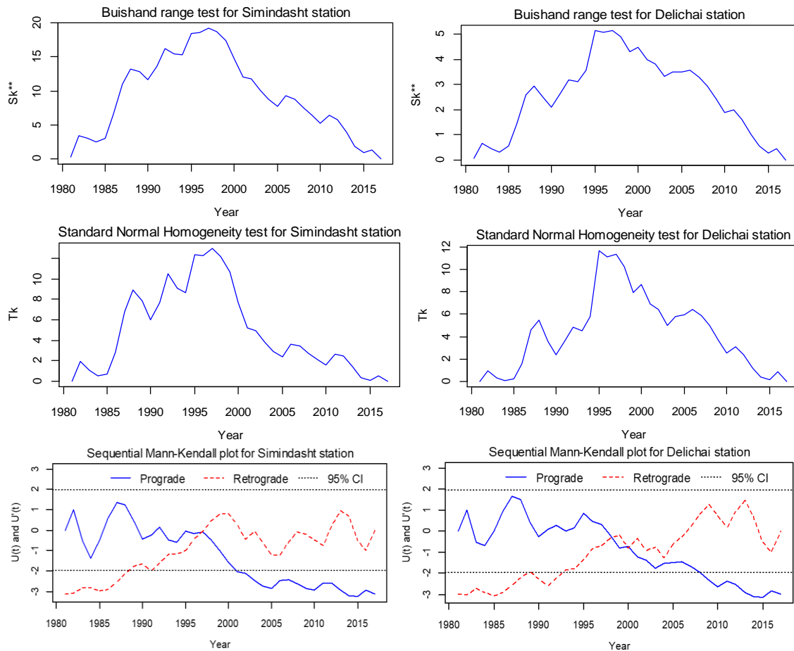
شکل ۳- نتایج آزمون‌های تعیین نقطه تغییر برای سری آبدهی متوسط سالانه در ایستگاه‌های هیدرومتری دلچای و سیمین‌دشت Figure 3- The results of different change point detection tests for the annual time series of discharge at the Delichai and Simindasht hydrometry stations
