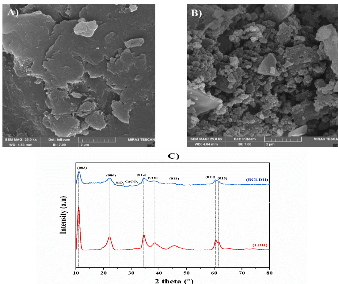
شکل ۲- تصاویر FE-SEM (A, B) و XRD (C) نمونه های پودری LDH و BCLDH.
