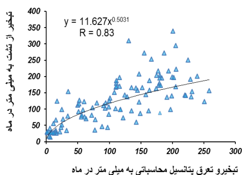
شکل ۲- مقایسه تبخیر و تعرق پتانسیل محاسباتی از روش بلانی-کریدل و تبخیر از تست
