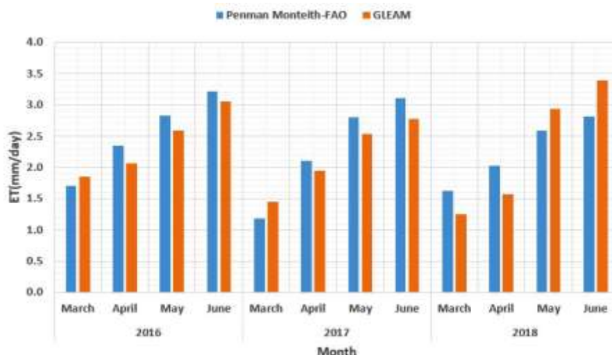
شکل ۵- مقایسه تغییرات تبخیرتعرق محاسبه شده حاصل از مدل GLEAM و پنمن مانیتث فائو برای ایستگاه رضوان Figure 5- Comparison of calculated evapotranspiration changes from GLEAM Model and FAO Penman-Monteith of the Rezvan station
