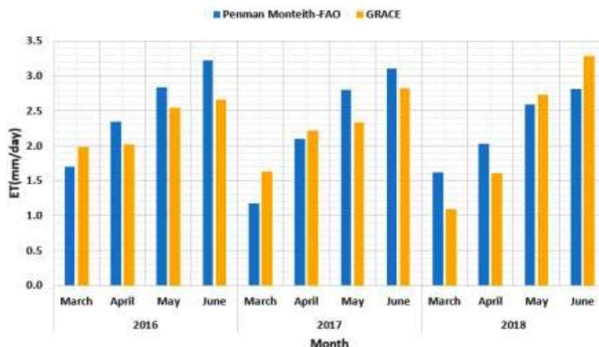
شکل ۷- مقایسه تغییرات تبخیرتقرق محاسبه شده حاصل از داده‌های ماهواره‌ای GRACE و رابطه پنمن مانیتث فائو برای ایستگاه رضوان Figure 7- Comparison of calculated evapotranspiration changes from GRACE and FAO Penman-Monteith satellite data of the Rezvan station
